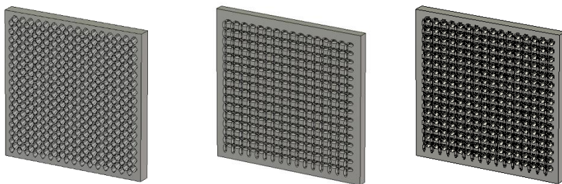
Рис.1. Модели антенных решеток из рупорных излучателей с ромбической, эллиптической и крестообразной формой излучающего раскрыва
