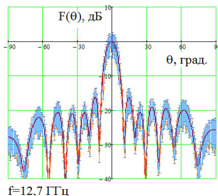
Рис.14. Диаграмма направленности с учетом амплитудных и фазовых ошибок для решетки из рупоров с эллиптическим раскрывом, в плоскости E на частоте 12,7 ГГц
