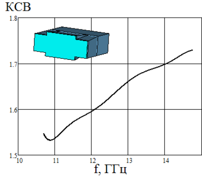
Рис.5. Зависимость КСВ от частоты излучателя, работающего в режиме передачи
