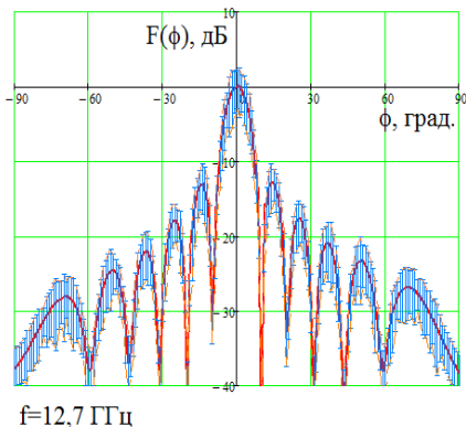
Рис.15. Диаграмма направленности с учетом амплитудных и фазовых ошибок для решетки из рупоров с эллиптическим раскрывом, в плоскости H на частоте 12,7 ГГц
