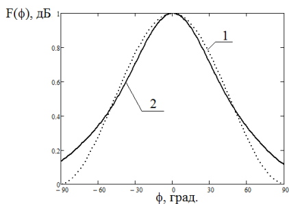
Рис.6. ДН излучателя в плоскости Н, рассчитанные аналитически (1) и численно (2) на частоте f=10,7 ГГц
