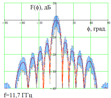
Рис.13. Диаграмма направленности с учетом амплитудных и фазовых ошибок для решетки из рупоров с эллиптическим раскрывом, в плоскости Н на частоте 11,7 ГГц
