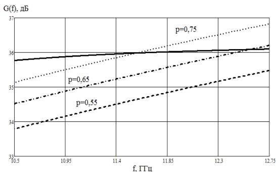
Рис.9. Зависимости коэффициента усиления от частоты антенной решеткой и зеркальной антенны при разной эффективности p
