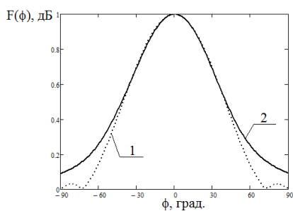
Рис.7. ДН излучателя в плоскости Н, рассчитанные аналитически (1) и численно (2) на частоте f=12,7 ГГц
