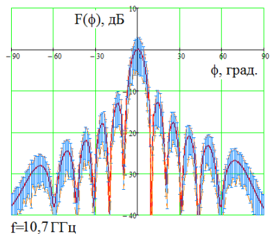
Рис.11. Диаграмма направленности с учетом амплитудных и фазовых ошибок для решетки из рупоров с эллиптическим раскрывом, в плоскости Н на частоте 10,7 ГГц
