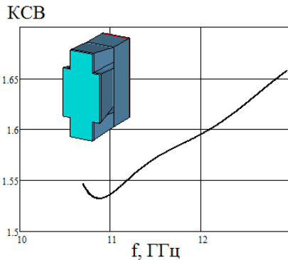
Рис.4. Зависимость КСВ от частоты излучателя, работающего в режиме приёма
