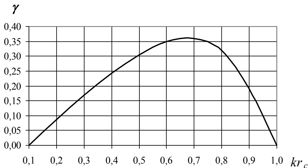
Рис. 5. Расчетная зависимость инкремента капиллярной неустойчивости от волнового числа (кривая Рэлея).
