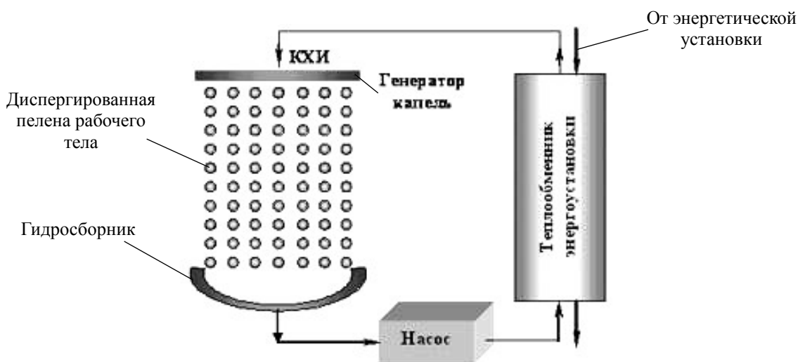
Рис. 3. Капельный холодильник-излучатель (КХИ).
