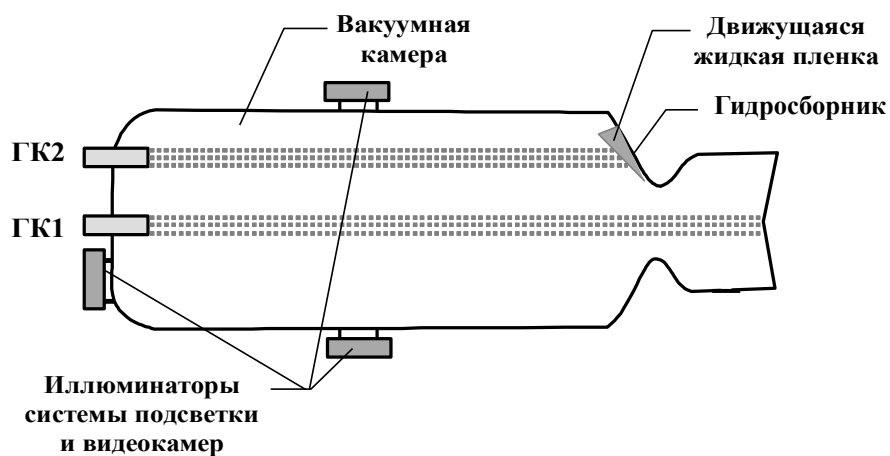
Рис. 9. Модель излучателя.
